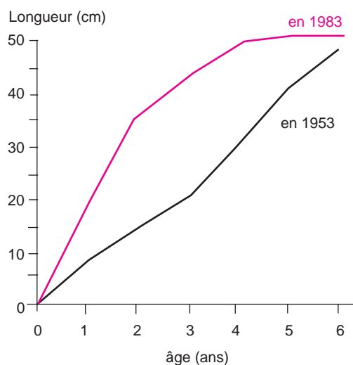
Figure 3. Croissance du corégone au lac Léman en 1953 et en 1983.
