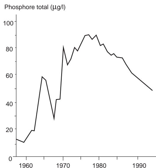
Figure 1. Evolution du taux de phosphore total dans le lac Léman.
