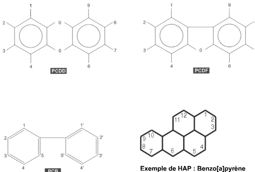
Figure 1. Structure des molécules PCDD/F, PCB et HAP.
