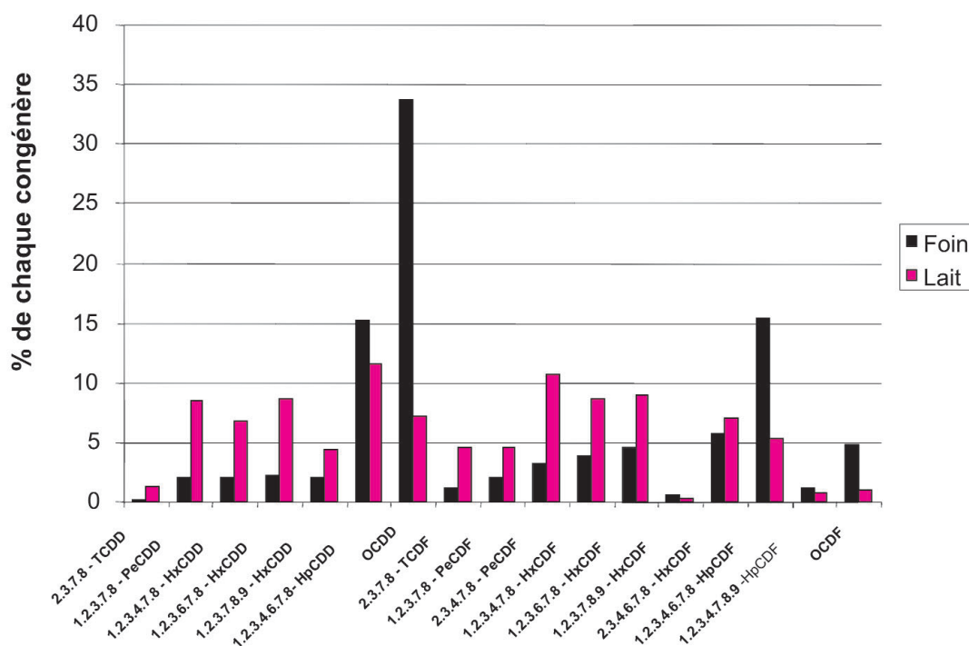
Figure 3. Comparaison des profils de PCDD/F entre le foin contaminé et le lait des chèvres ayant consommé ce foin.
