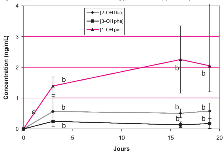
Figure 2. Evolution des concentrations de métabolites hydroxylés dans le lait suite à l'ingestion quotidienne de sol contaminé (500g/j) en fluorène, pyrène et phénanthrène.
